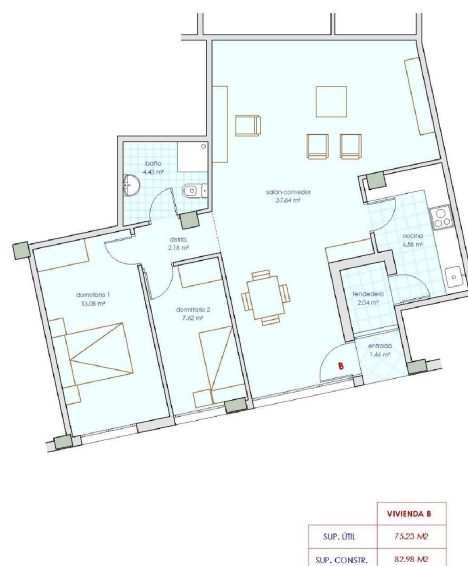
ACONDICIONAMIENTO DE LOCAL PARA 4 VIVIENDAS VIVIENDA TIPO B ESCALA 1/75
